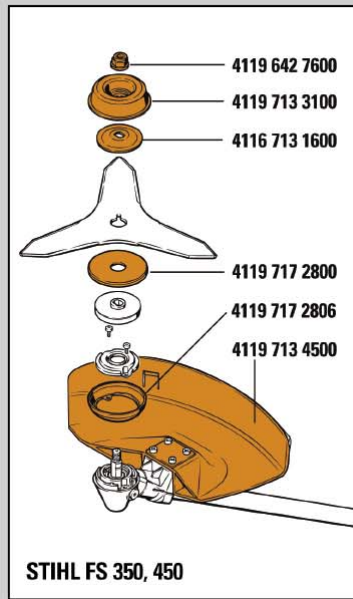
STIHL FS 350, 450
